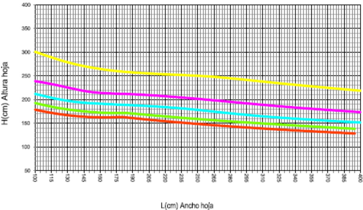
DIMENSIONES MÁXIMAS
