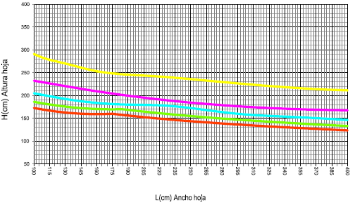
DIMENSIONES MÁXIMAS
